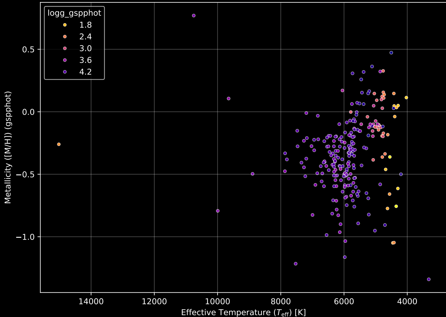
GALAH DR4 Field: [7225] Stellar Population Parameters (n= 242)
