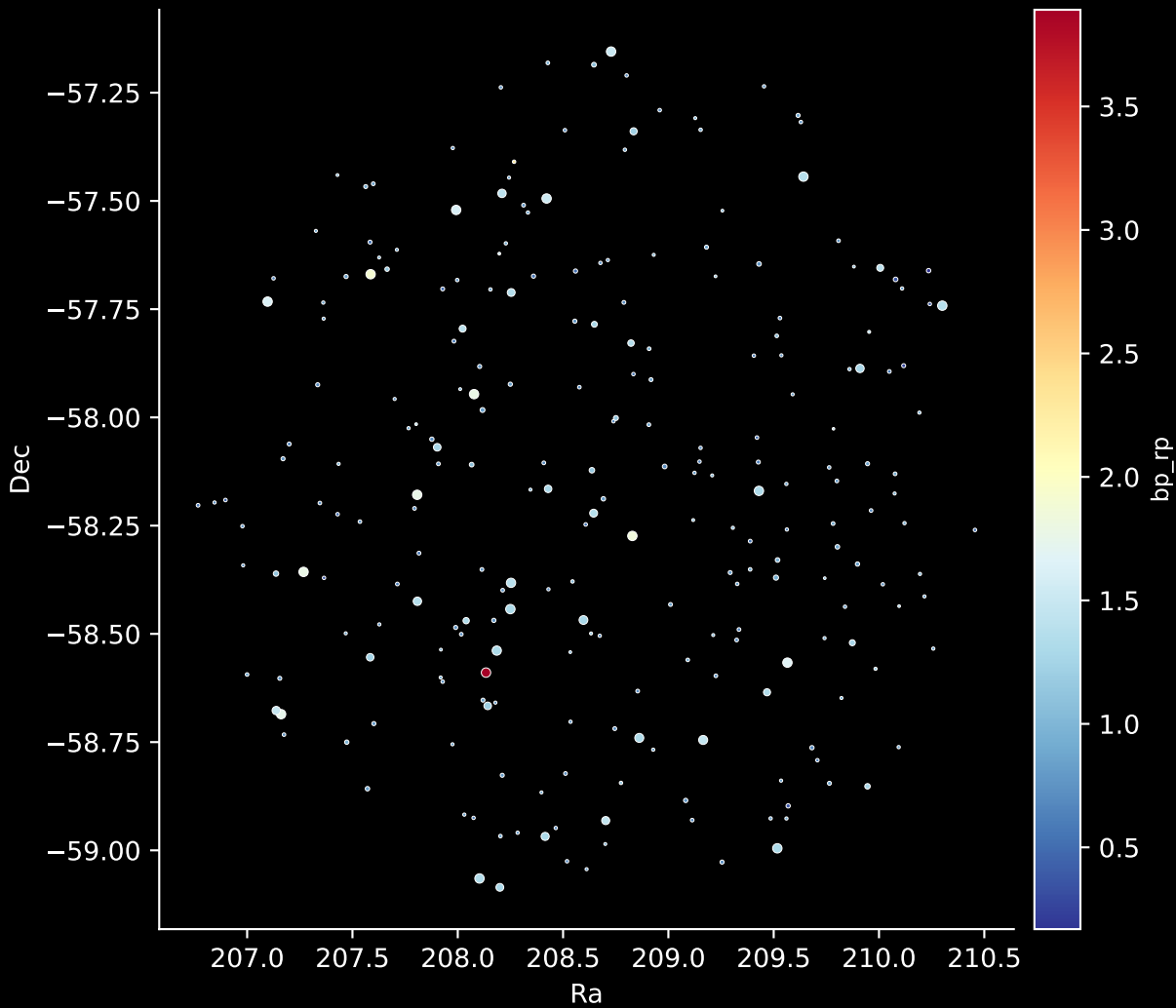
GALAH DR4 Field: [7225] Stars: 242
