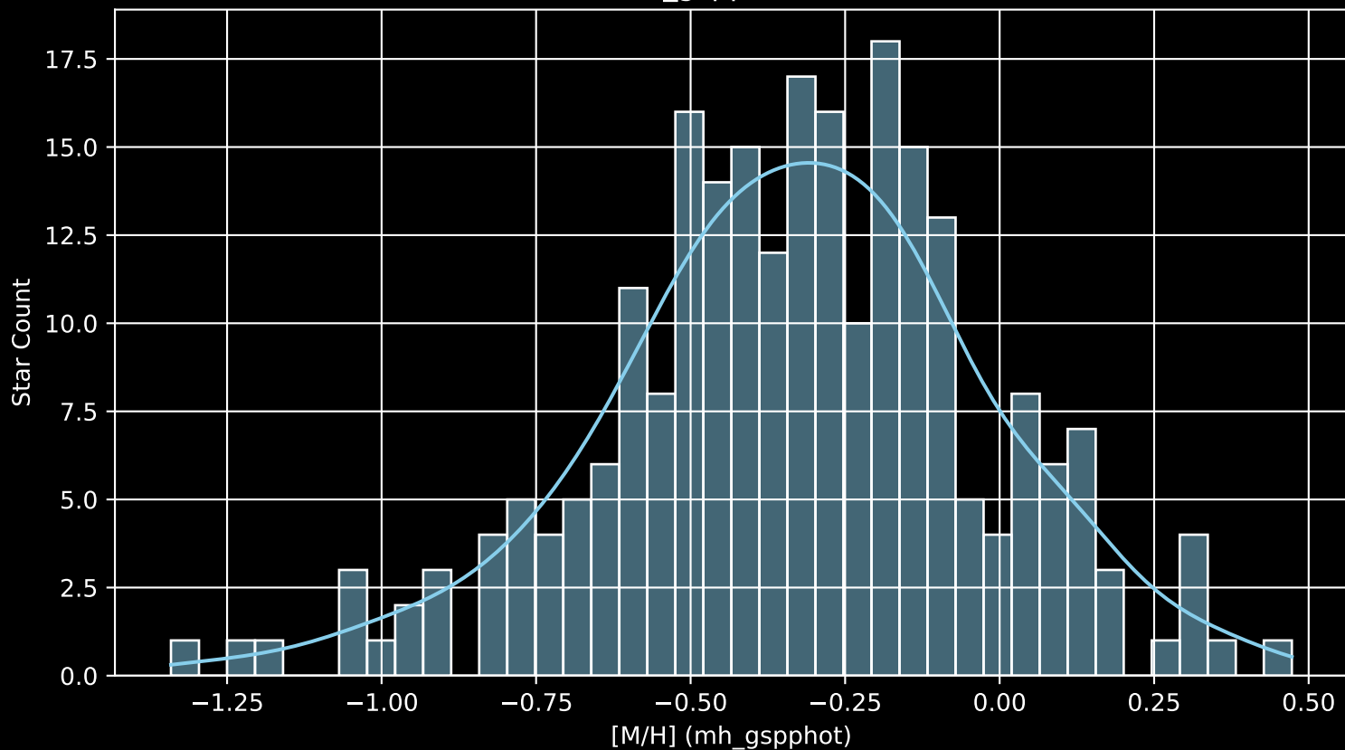
GALAH DR4 Field: [7225] [M/H] (mh_gspphot) (n= 241)
